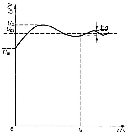
图3 发电机空载阶跃响应曲线
