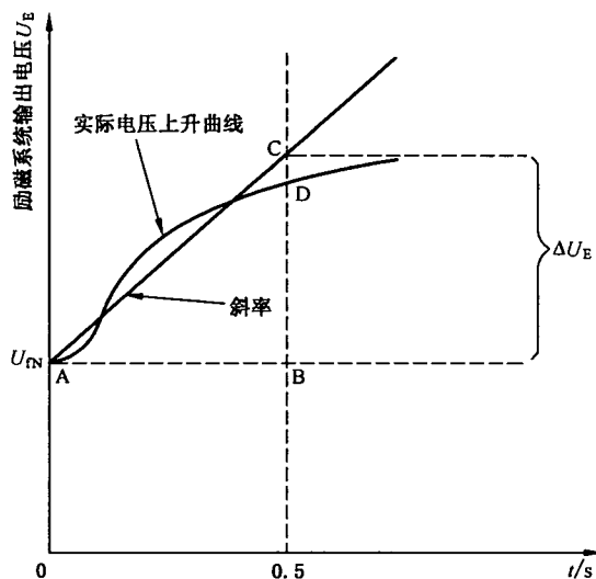
图2 励磁系统标称响应 V_E 的确定
